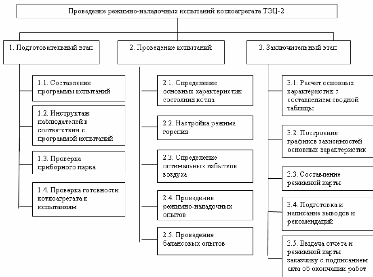
Рис. 2. Структурная декомпозиция работ режимно-наладочных испытаний
