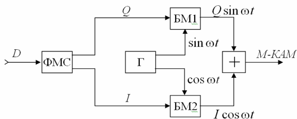
Рис. 1. Схема получения многопозиционной модуляции
