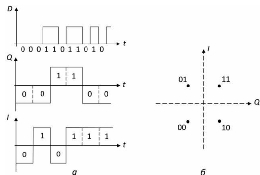
Рис. 2. Осциллограммы сигналов
